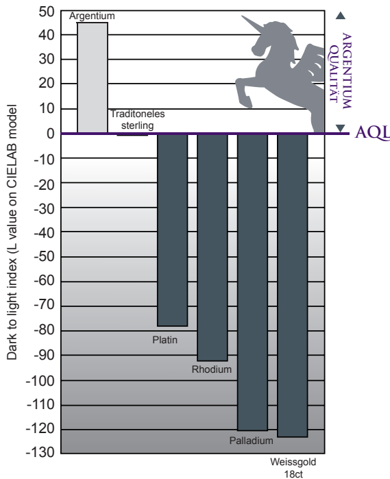
Glanz- Diagramm (Hell/Dunkel-Messung L- Wert)
